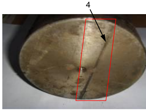
图 8a 柱塞端部磨损示意图
